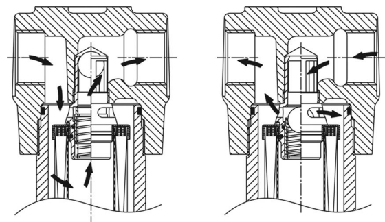
Filtration mode
